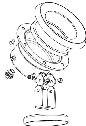
水下燈結構圖
