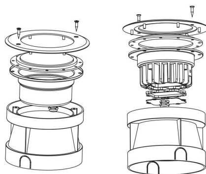
LED 水下埋地燈結構圖
