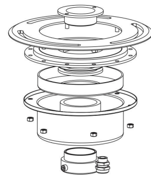
不銹鋼噴泉燈結構圖
